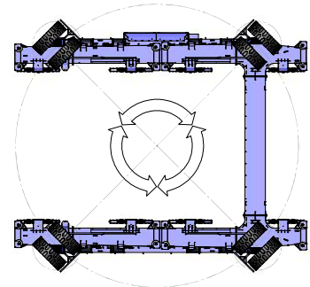
Konzentrische Lenkung
