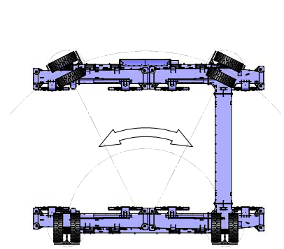
Allradlenkung
