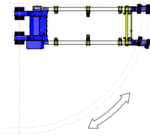
Diagonallenkung
