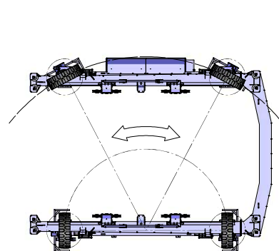
Allradlenkung
