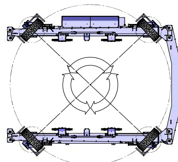
Konzentrische Lenkung
