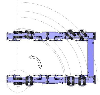
Lenkung der Hinterräder
