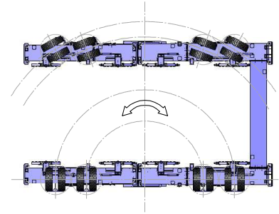
Konzentrische Lenkung
