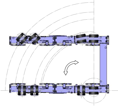
Lenkung der Vorderräder
