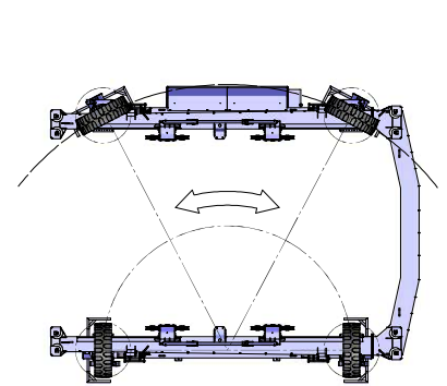
Ruedas todas directrices
