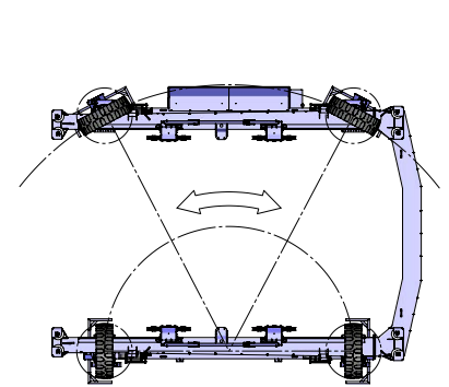
Allradlenkung
