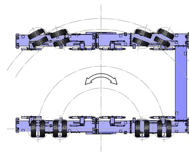
Rotation sur place
